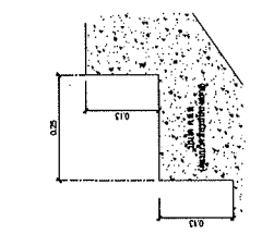
แบบค้ำยันได้ 1:100
