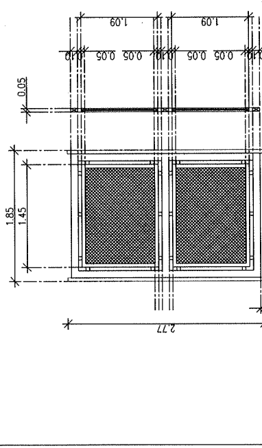
แบบขยายประตู - 1
